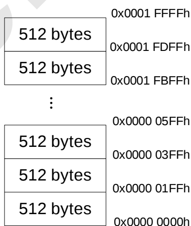
SC32M15X 系列 128 Kbytes APROM Sector 分区示意
